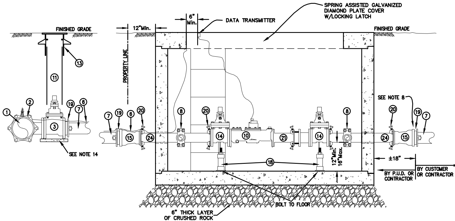
ELEVATION
