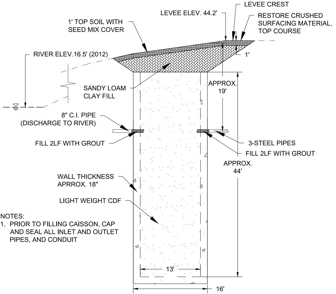
RANNEY WELL CAISSON (SCHEMATIC) N.T.S.
